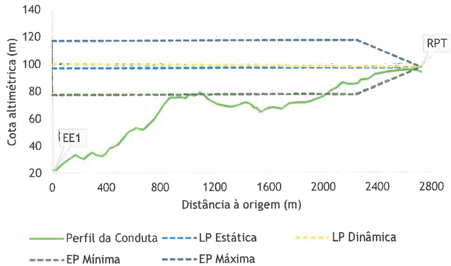
Figura 8.23. Perfil teórico das envolventes de pressão extrema no sistema EE1-RPT - Sol. A
