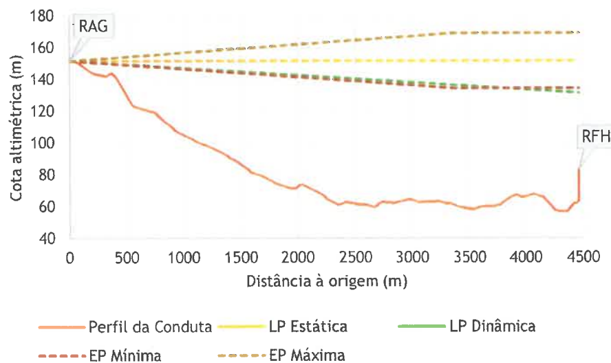
Figura 8.31. Perfil teórico das envolventes de pressão extrema no sistema RAG-RFH - Sol. B
