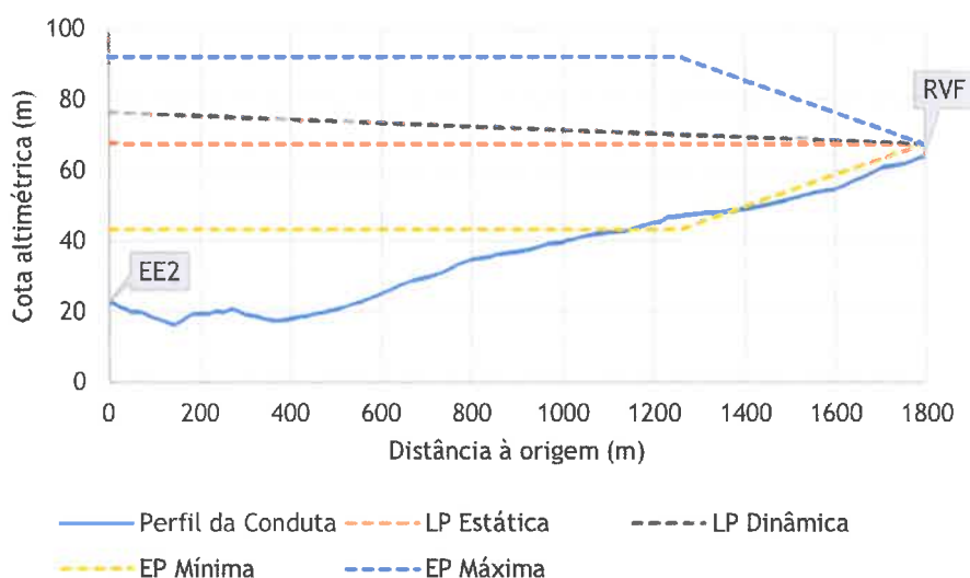
Figura 8.34. Perfil teórico das envolventes de pressão extrema no sistema EE2-RVF - Sol. C
