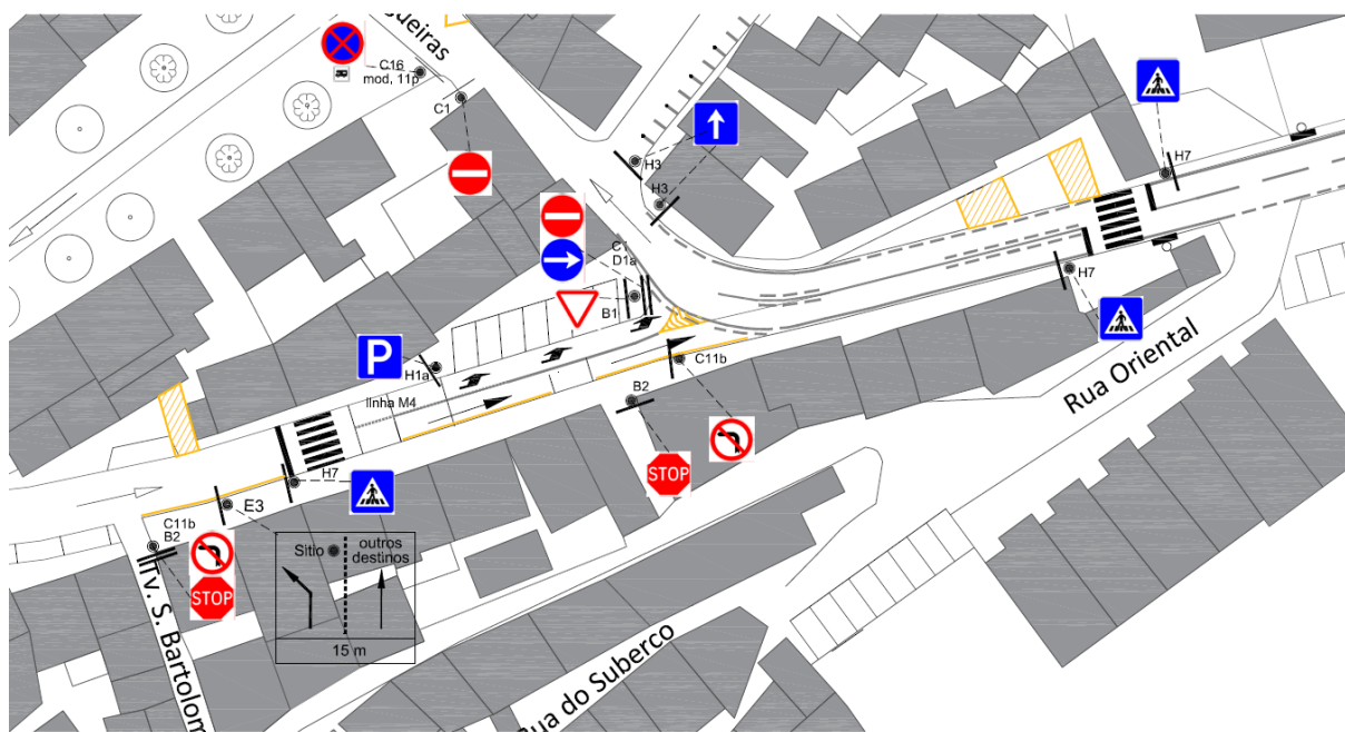
Extrato da planta com a proposta de alteração ao plano de trânsito, sem escala
