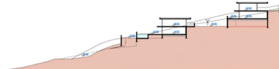
CORTE GH
