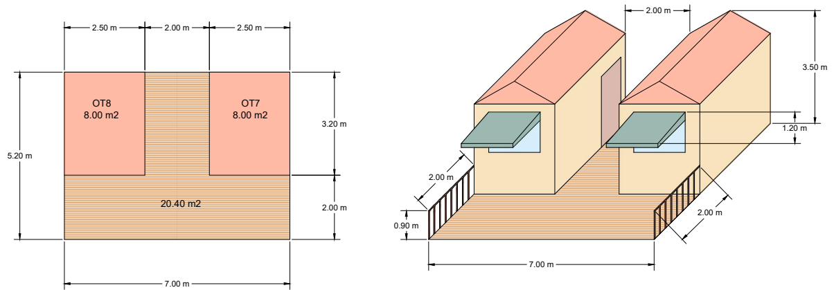
Esquema de implantação da Ocupação Temporária do Domínio Público Marítimo (OT7 e OT8) (Solução esquemática em caso de partilha de estrado)
