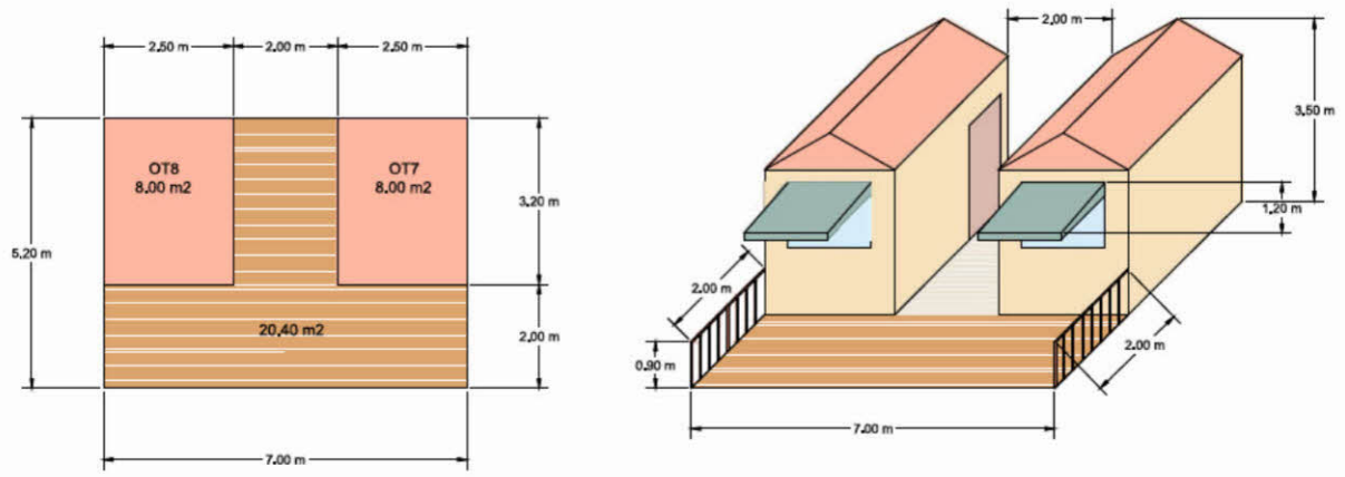
Esquema de implantação da Ocupação Temporária do Domínio Público Marítimo (OT7 e OT8) (Solução esquemática em caso de partilha de estrada)
