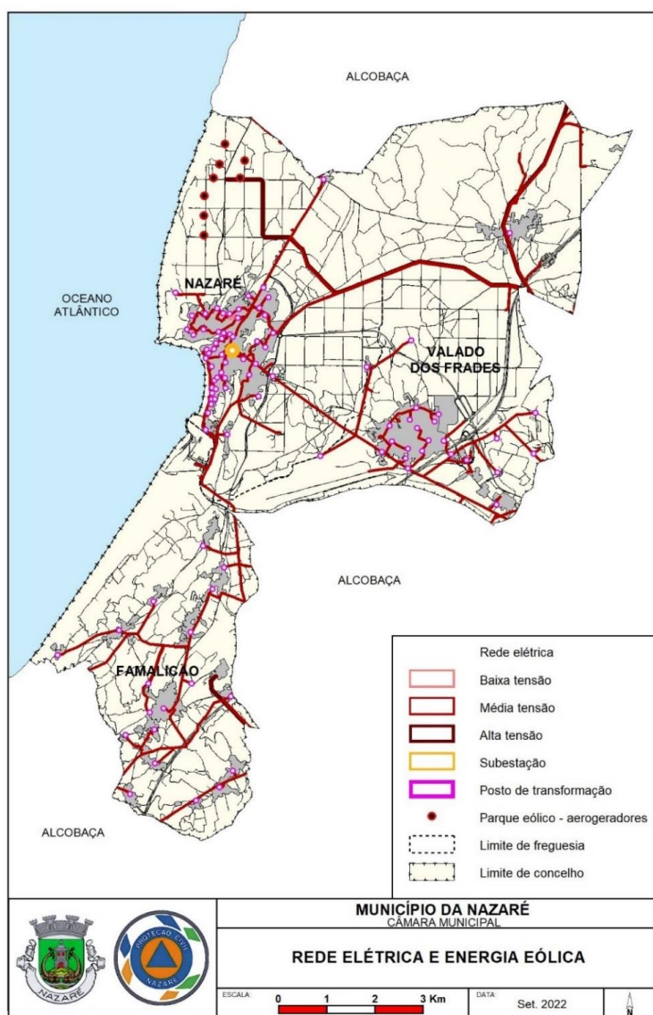
Figura 10 – Rede de transporte e distribuição de energia elétrica
