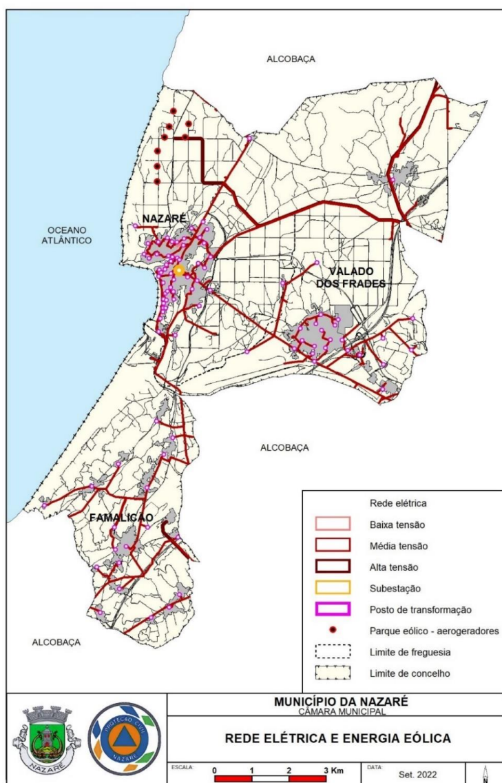
Mapa 6 – Rede de transporte e distribuição de energia elétrica
