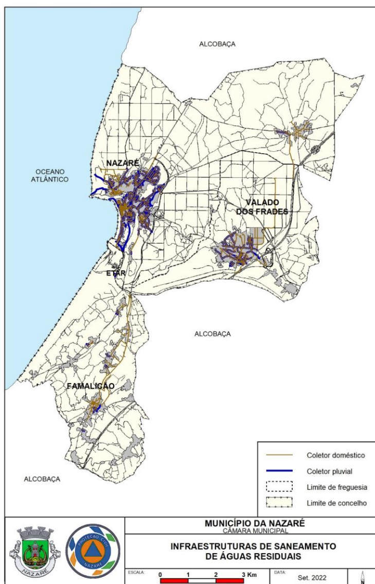
Mapa 5 – Infraestruturas de Saneamento de Águas Residuais
