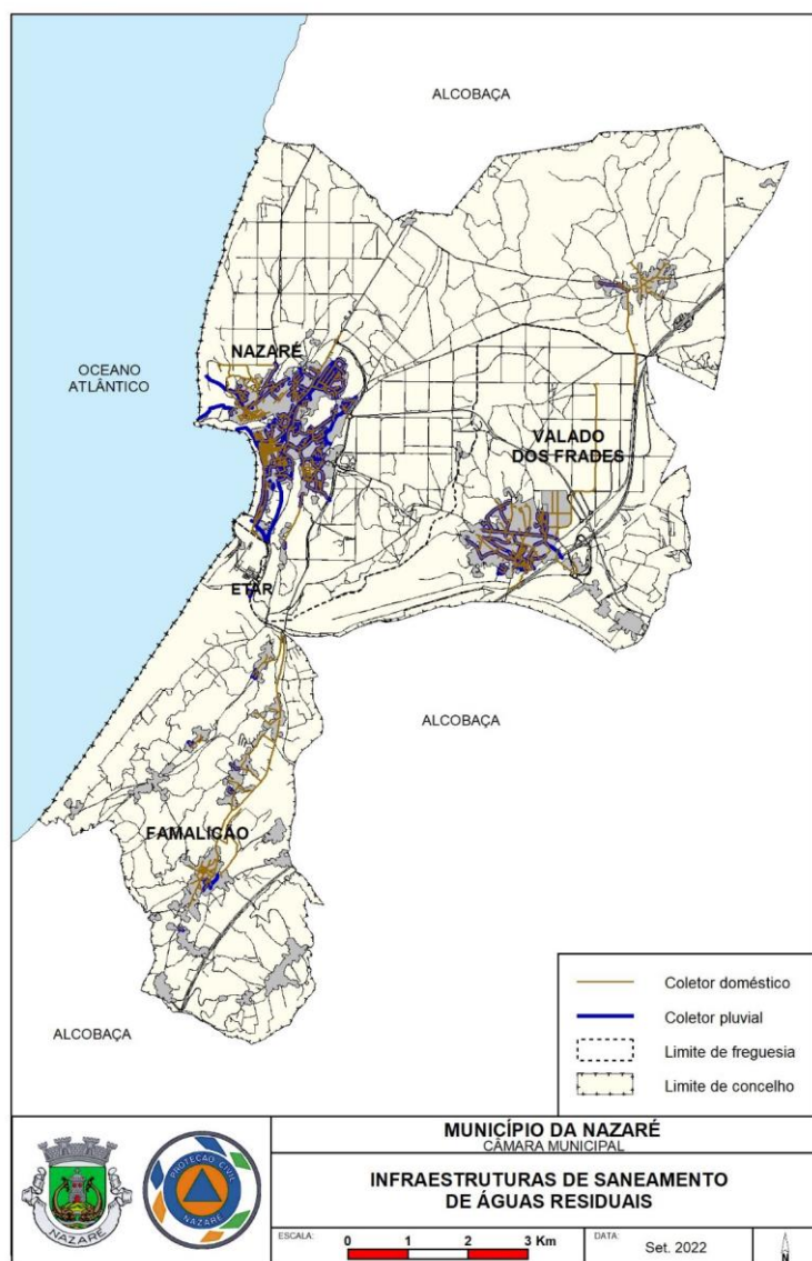
Figura 9 – Infraestruturas de Saneamento de Águas Residuais
