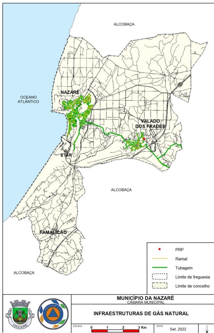
Mapa 7 – Rede de distribuição de Gás Natural
