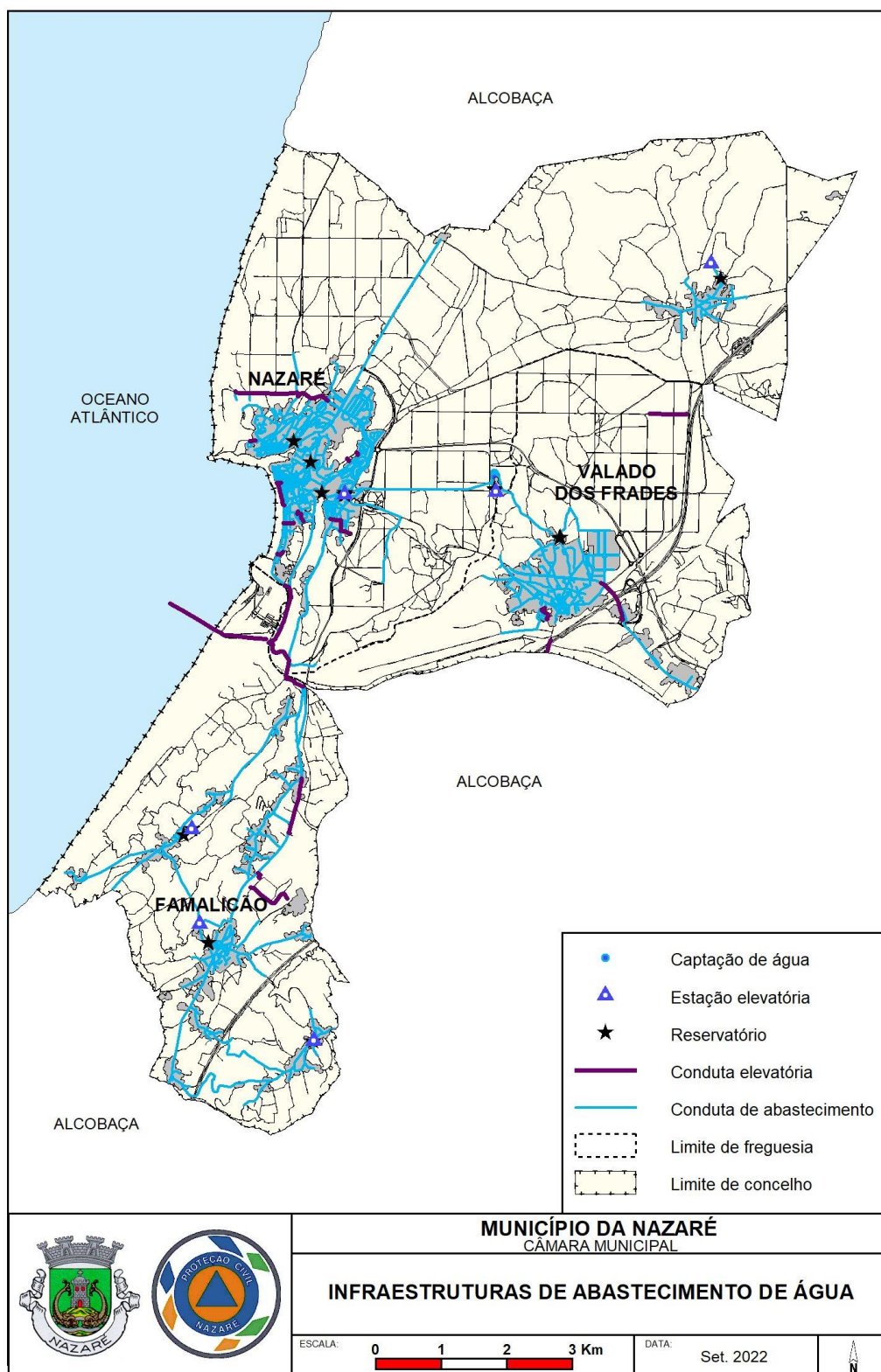
Figura 8 – Infraestruturas de Abastecimento de Água
